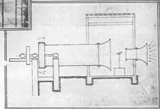
Dibujo esquemático de la cámara de experimentación.
