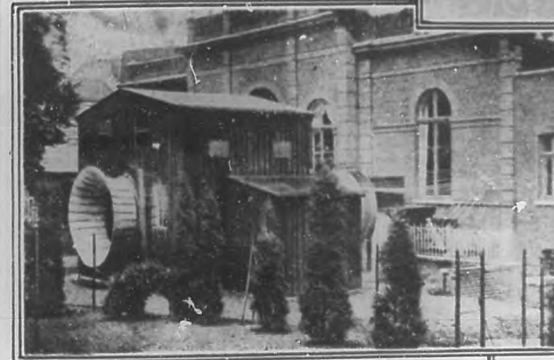
Instalación "Junkers" de corriente de canal para examinar modelos de aviones.
